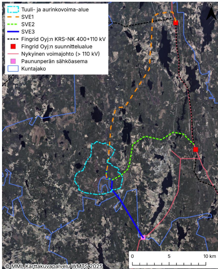
Kuva 10. Hankealue ja suunnitellut sähkönsiirtoreitit ilmakuvassa.
