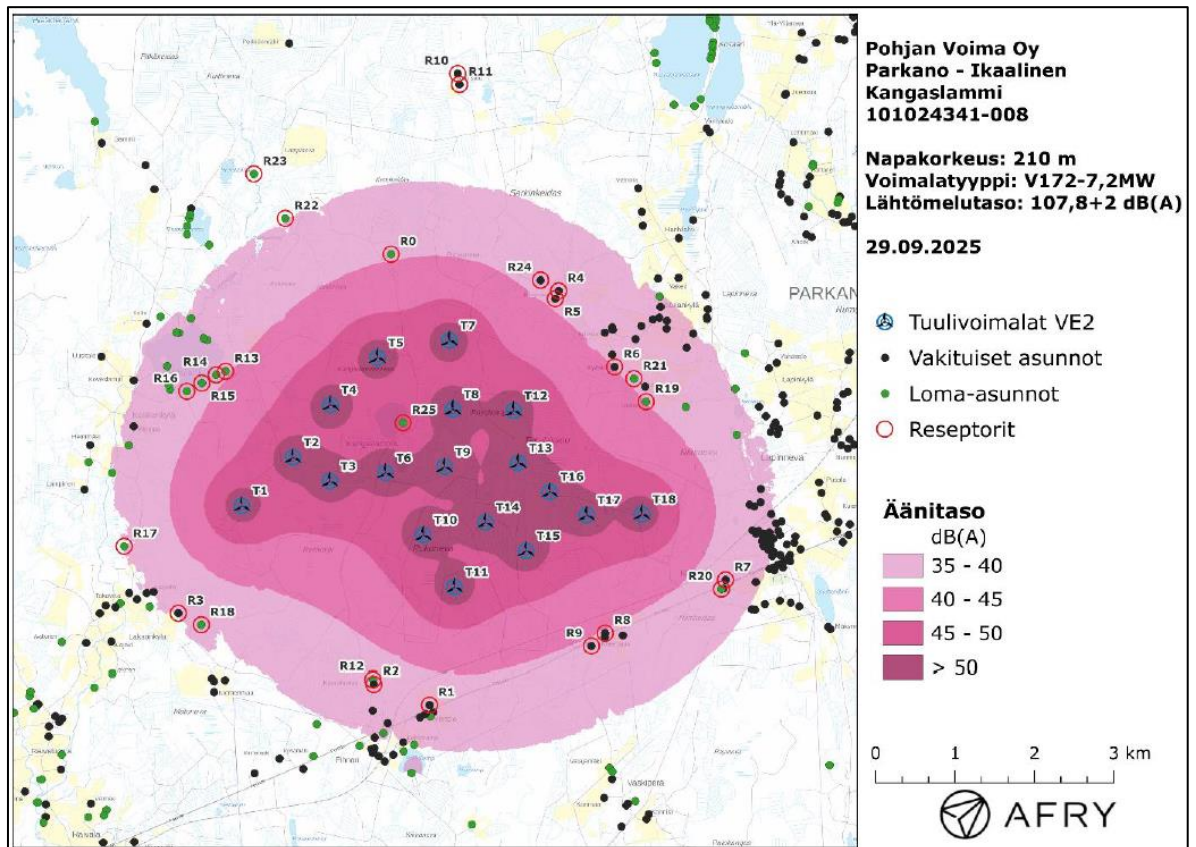
Kuva 66 Keskiäänitasot LAeq Kangaslammin toteutusvaihtoehdolla VE2
