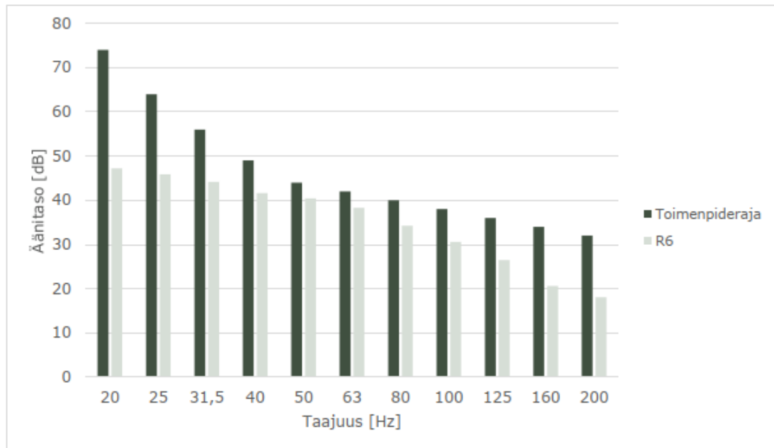
Kuva 67. Matalataajuisen sisämelun tasot reseptorin R6 kohdalla tuulivoimavaihtoehdossa TV2 (Afry Finland Oy).
