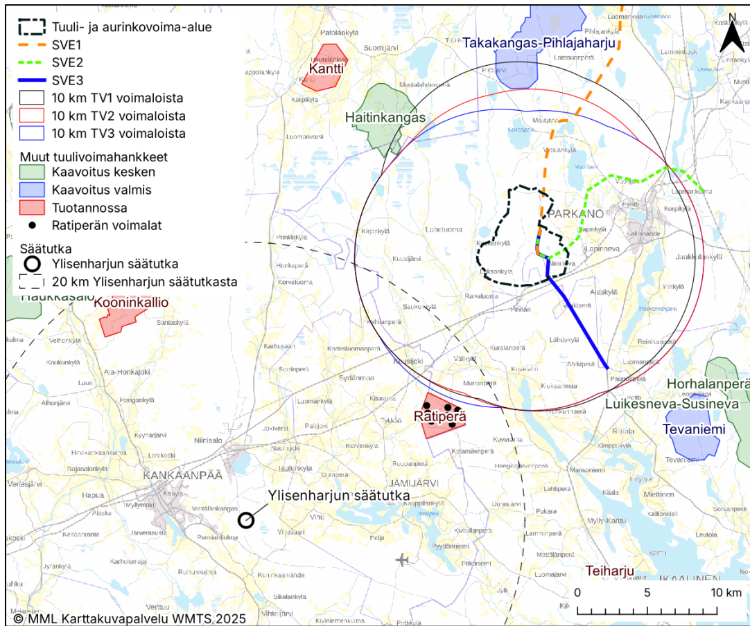
Kuva 70. Hankealueen sijoittuminen suhteessa Ylisenharjun säätutkaan.
