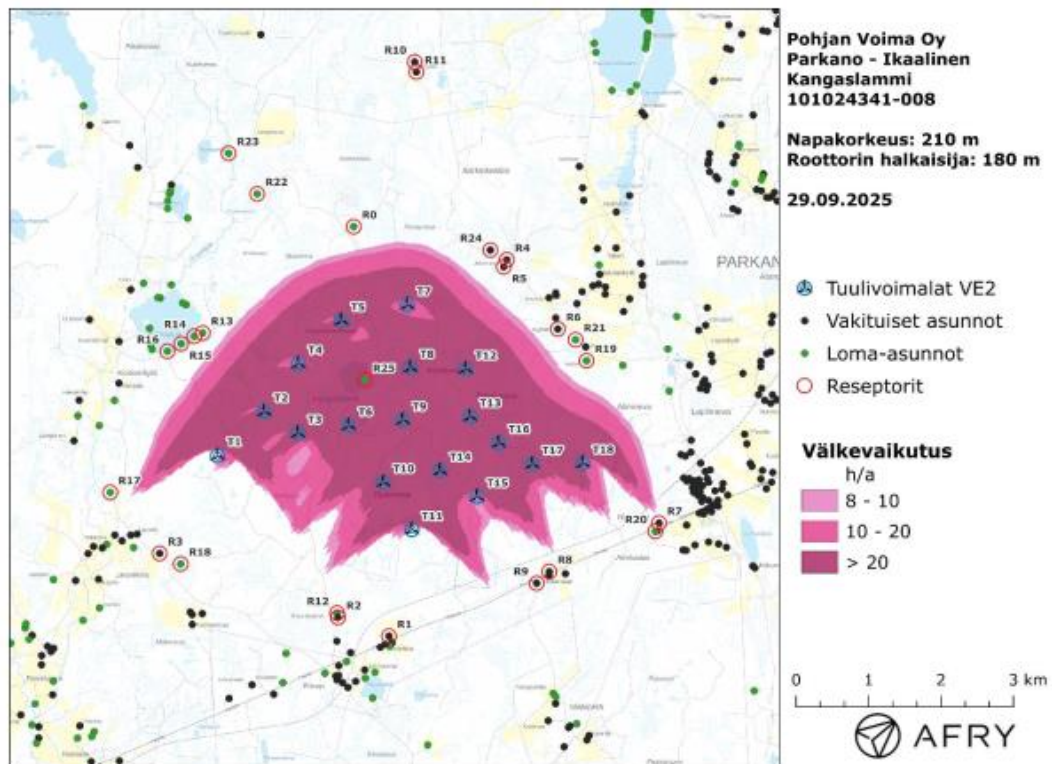
Kuva 68 Tuulivoimaloiden aiheuttama välnketuntien määrä ilman puuston vaikutusta tuulivoimavaihtoehdossa TV2 (Afrý Finland Oy, 2025b).
