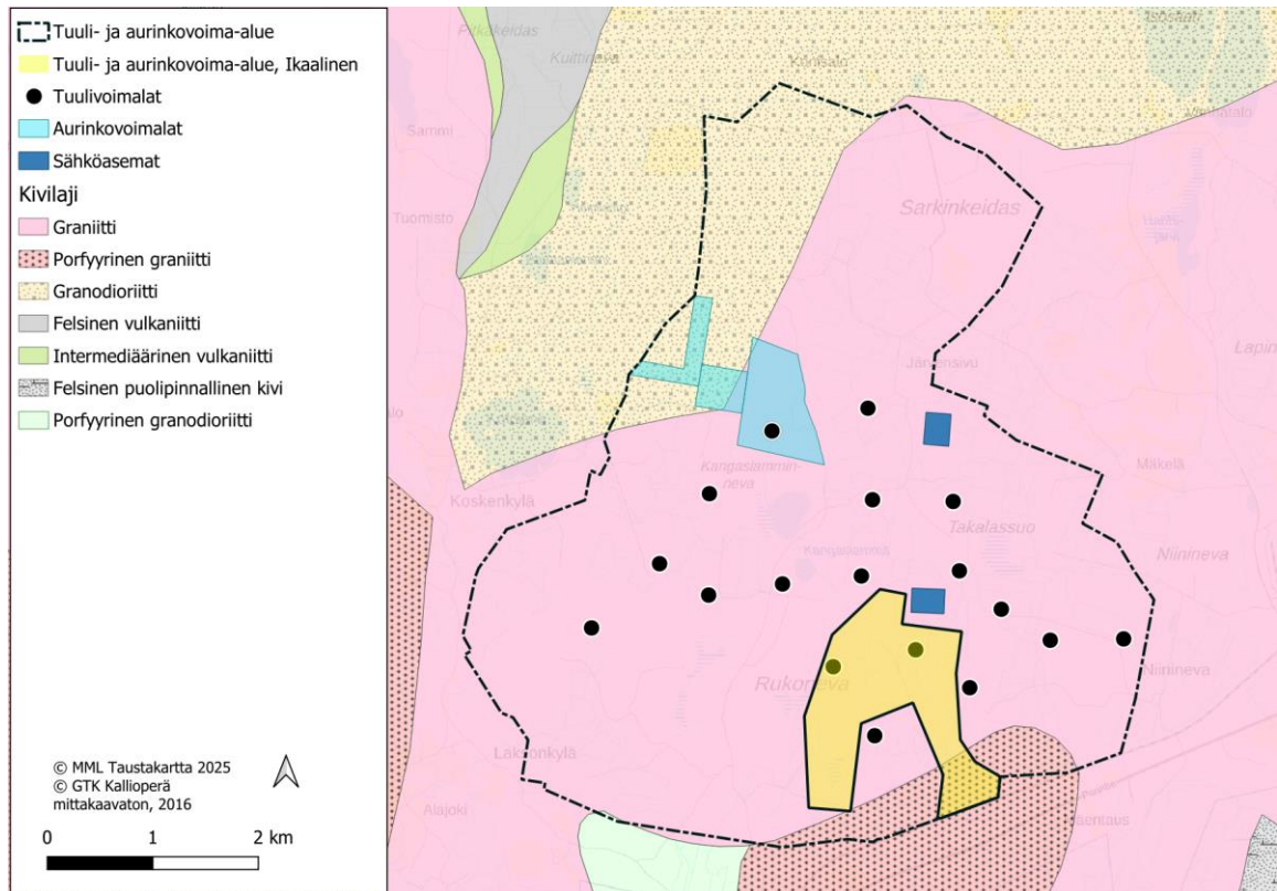
Kuva 14. Tuuli- ja aurinkovoima-alueen kallioperä. (GTK 2016)
