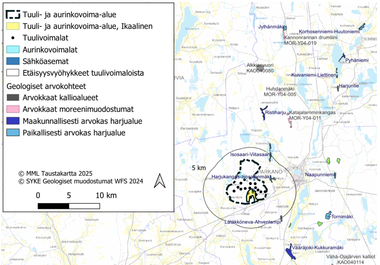
Kuva 17. Hankealueen ympäristön geologisesti arvokkaat kohteet. (Suomen ympäristökeskus 2024, Pirkanmaan liitto 2015)
