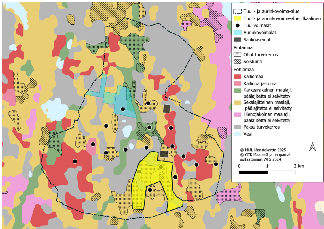
Kuva 15. Tuuli- ja aurinkovoima-alueen maaperä. (GTK 2024)
