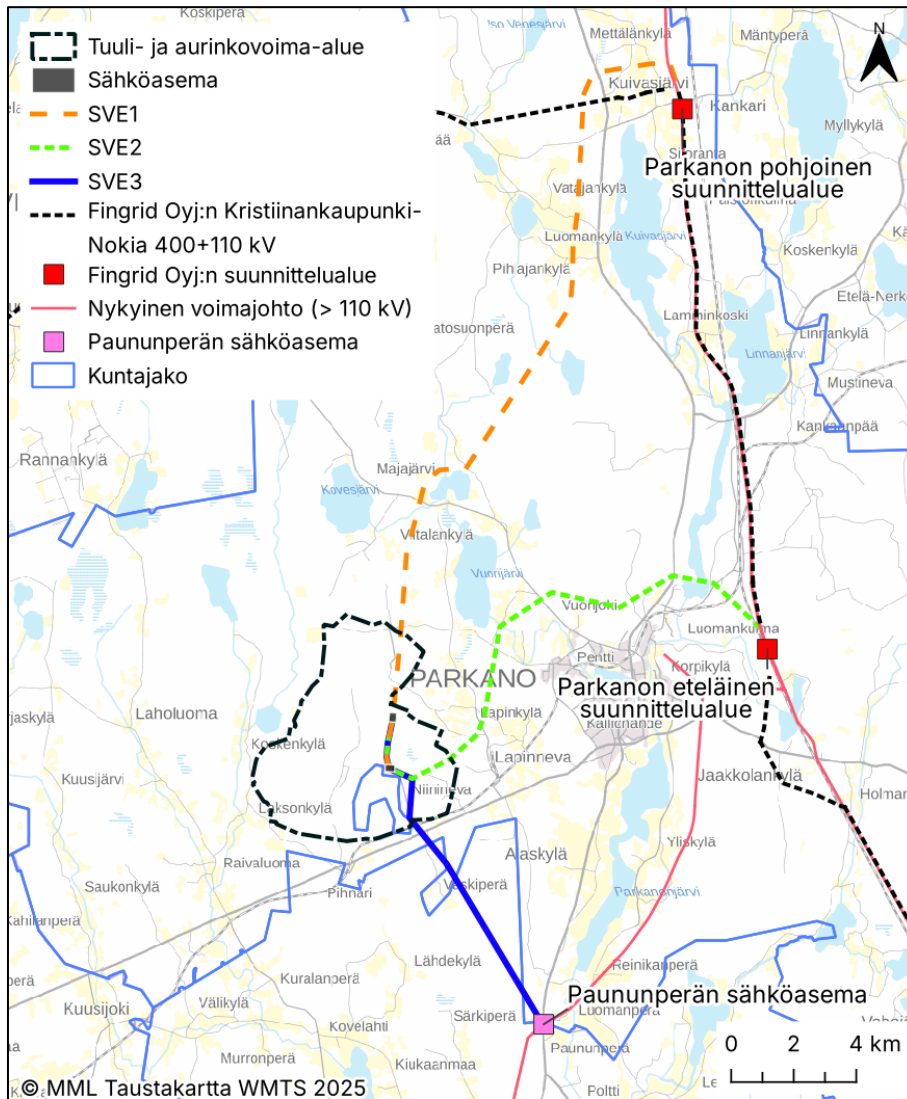
Kuva 2. Osayleiskaava-alue ja sähkönsiirron vaihtoehdot
