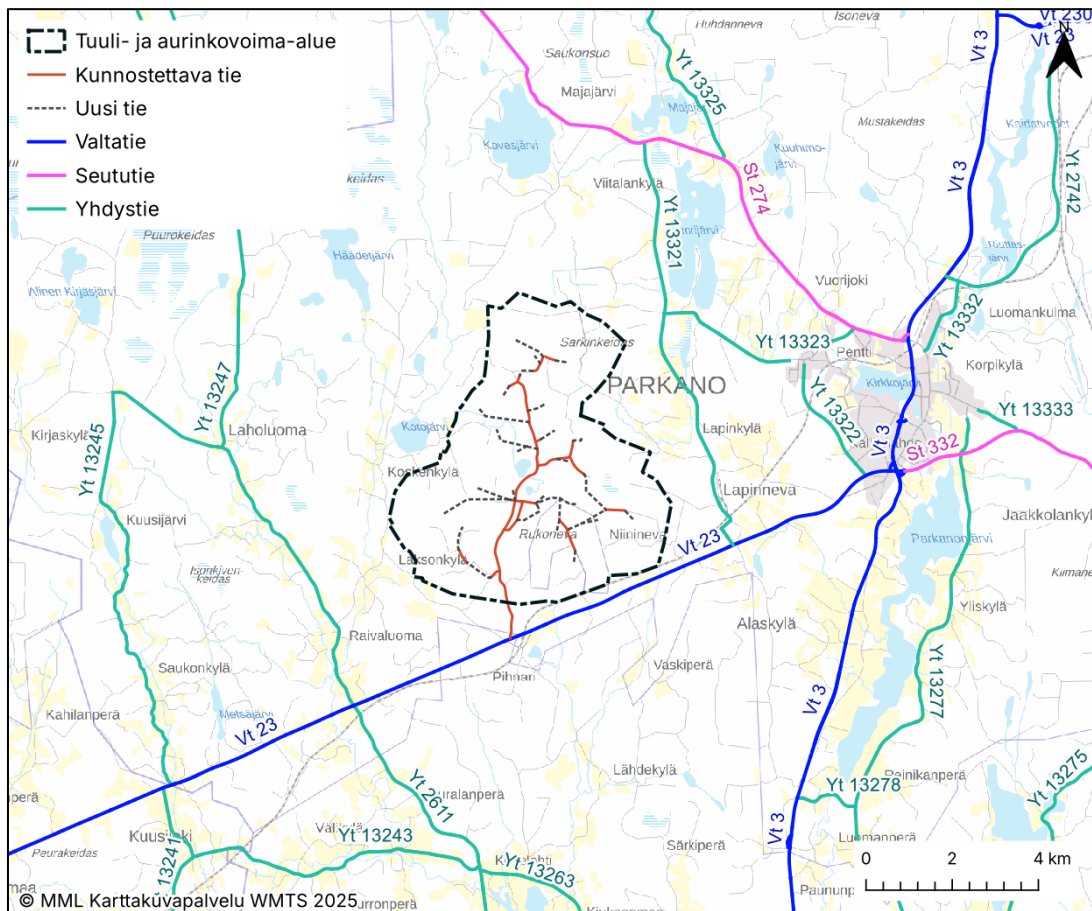
Kuva 40. Hankealuetta ympäröivä tieverkko ja hankealueelle rakennettavat uudet sekä parannettavat tiet.
