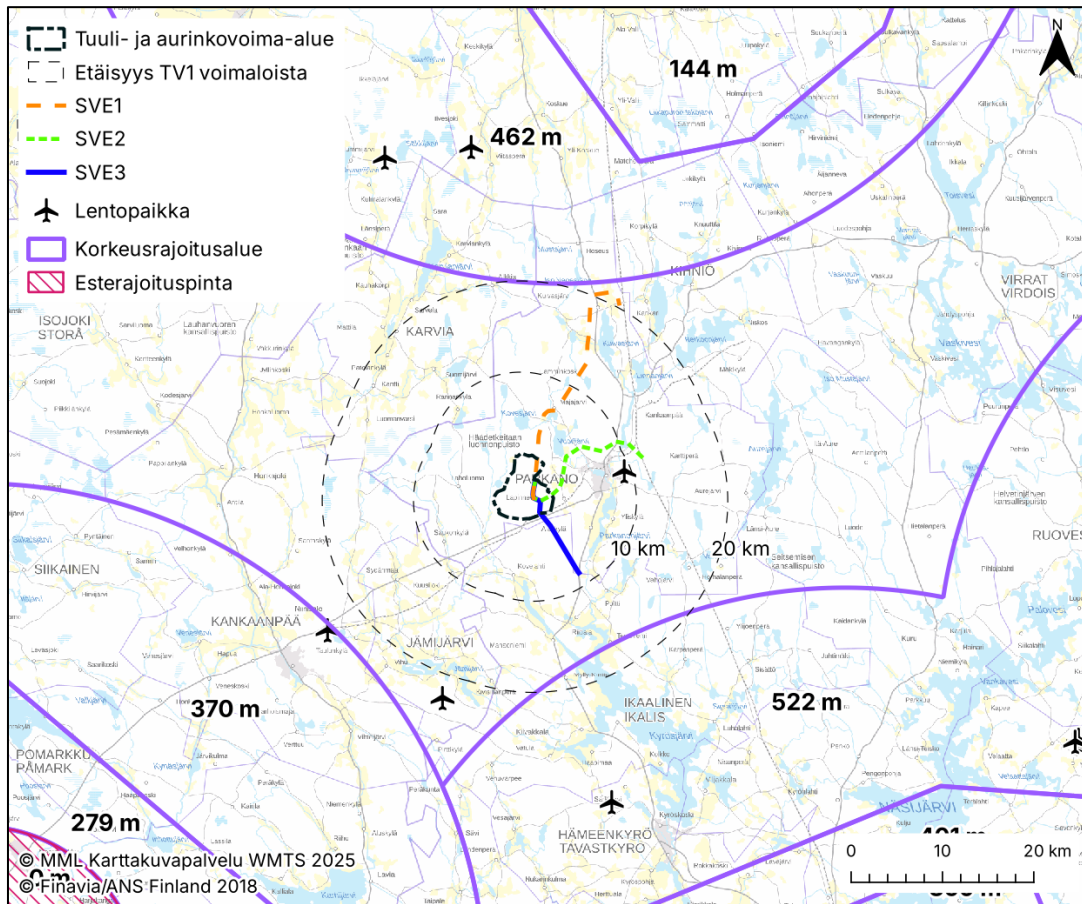
Kuva 69. Lentoestealueet hankealueen läheisyydessä.
