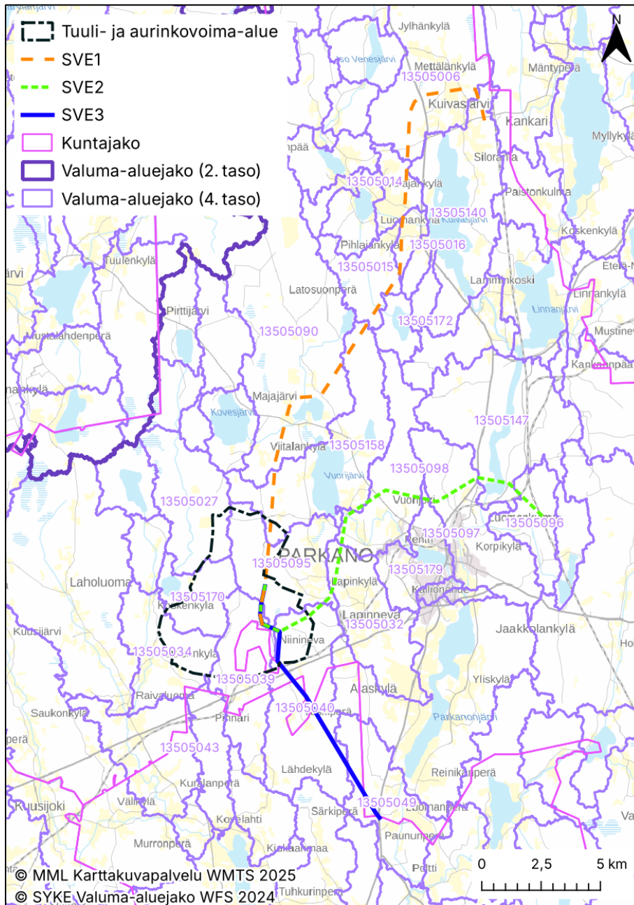
Kuva 19. Hankealueen sijainti valuma-alueilla (Suomen ympäristökeskus 2024).
