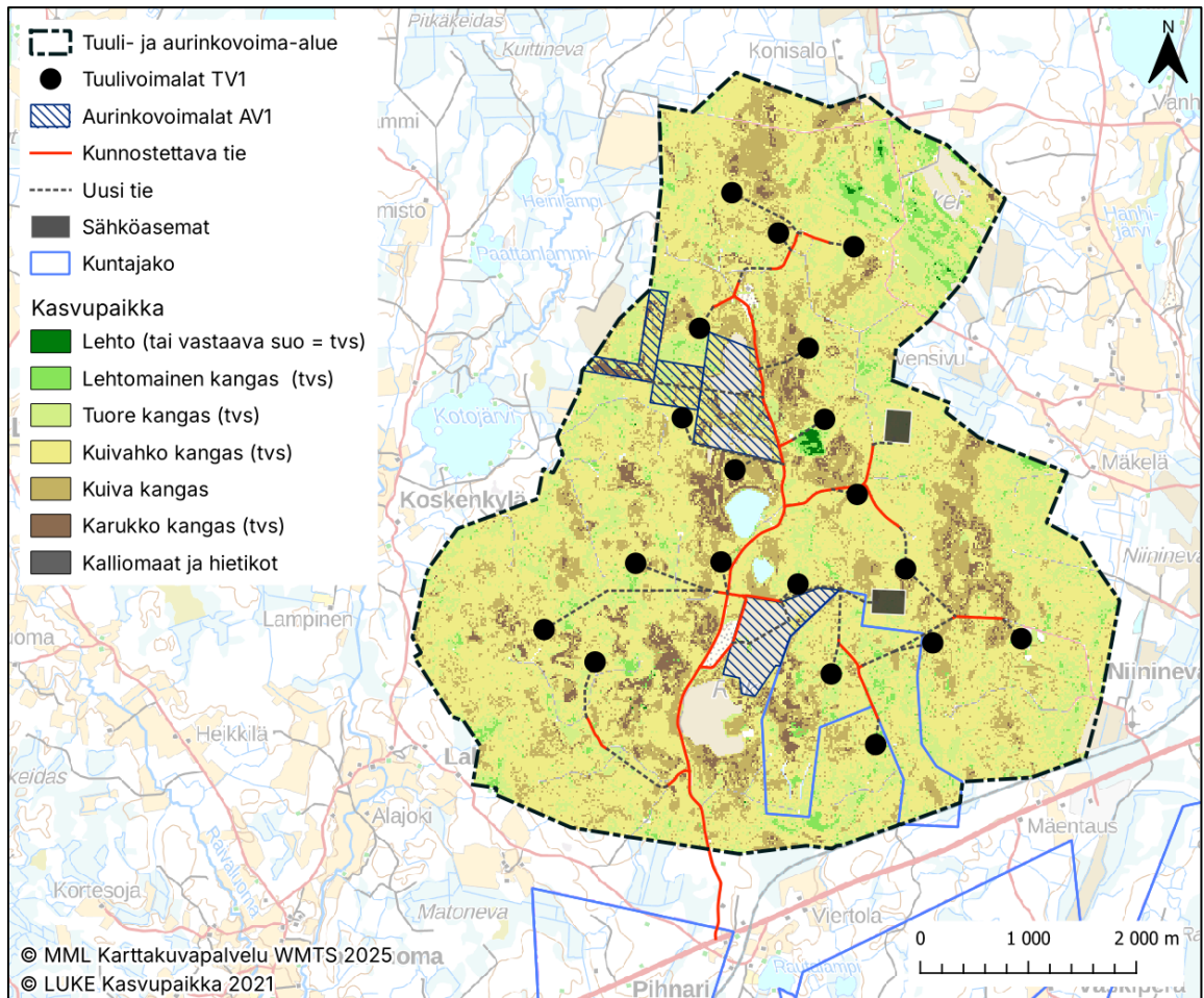
Kuva 22. Hankealueen kasvupaikkatyypit. (Luonnonvarakeskus 2021)
