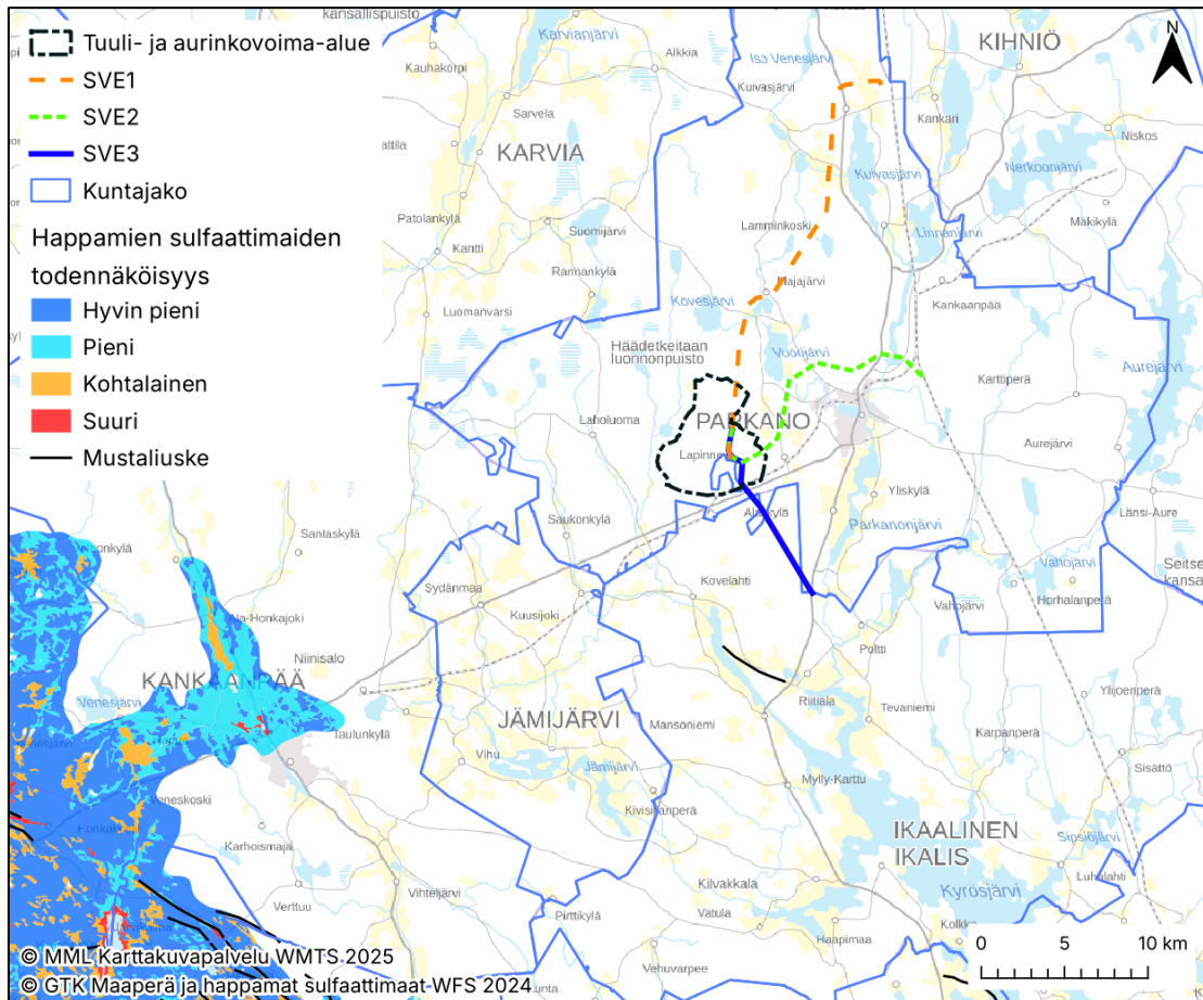
Kuva 16. Happamat sulfaattimaat hankealueen läheisyydessä (Geologian tutkimuskeskus 2024).
