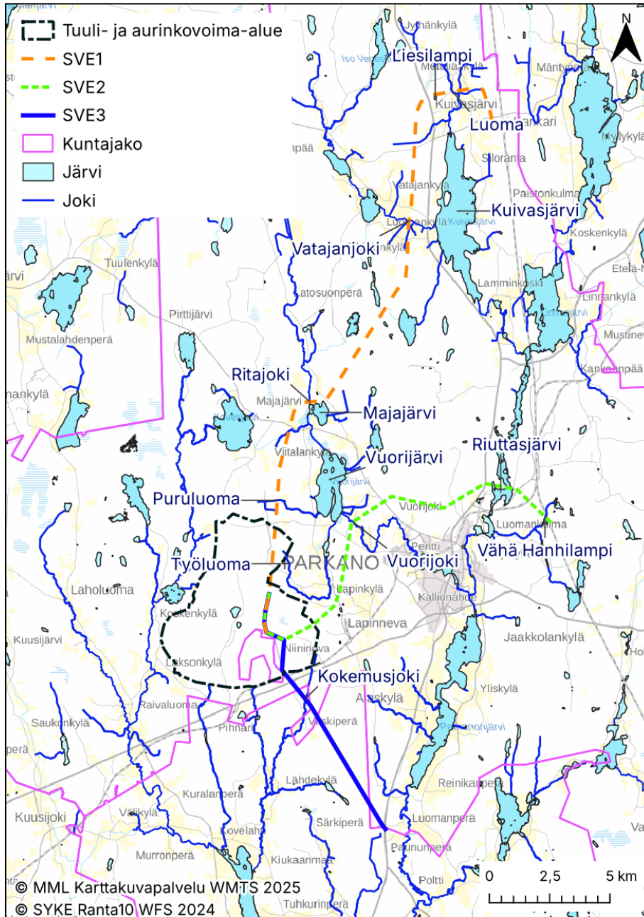
Kuva 20. Kangaslammin hankealueen pintavedet. (Suomen ympäristökeskus 2024)
