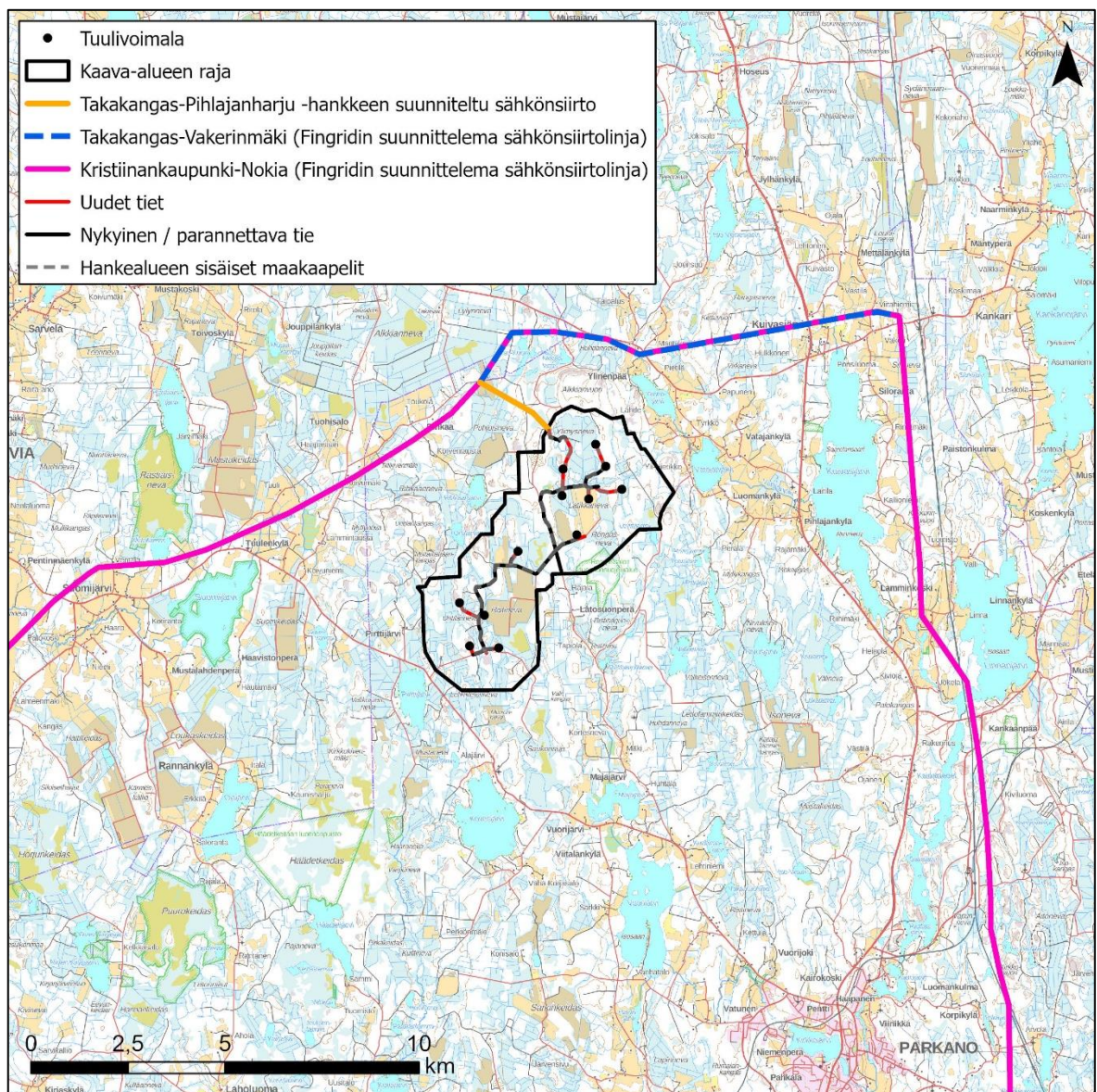
Kuva 1.4. Hankkeen ulkoinen sähkönsiirto, voimalasijoittelu, maakaapelilinjaukset ja suunniteltu tiestö.
