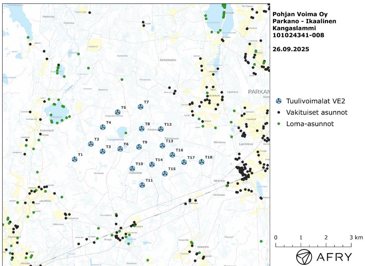
Kuva 1-1: Tuulivoimaloiden sijainnit Kangaslammin toteutusvaihtoehdolla VE2.
