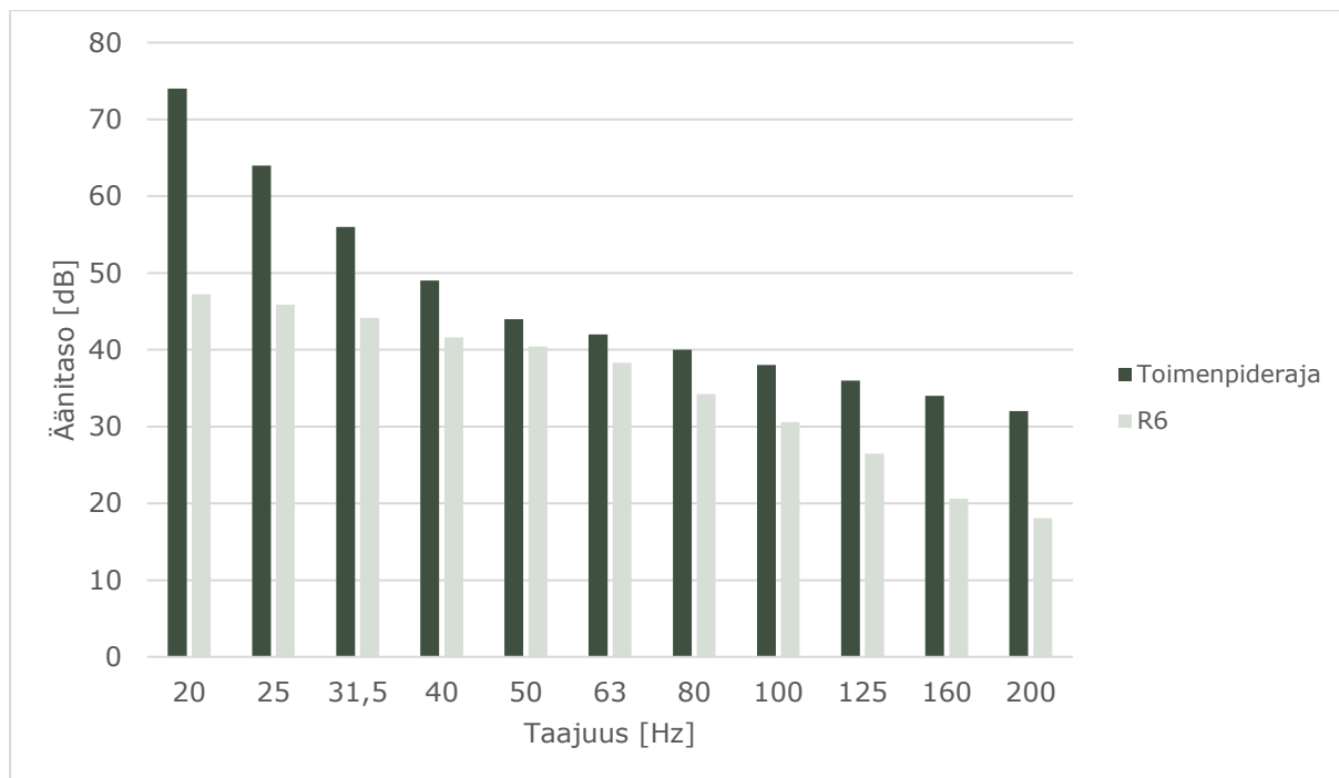
Kuva 3-3: Matalataajuisen sisämelun tasot reseptorin R6 kohdalla.
