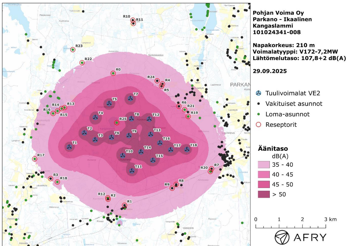
Kuva 3-2: Keskiäänitasot L_{Aeq} Kangaslammin toteutusvaihtoehdolla VE2.
