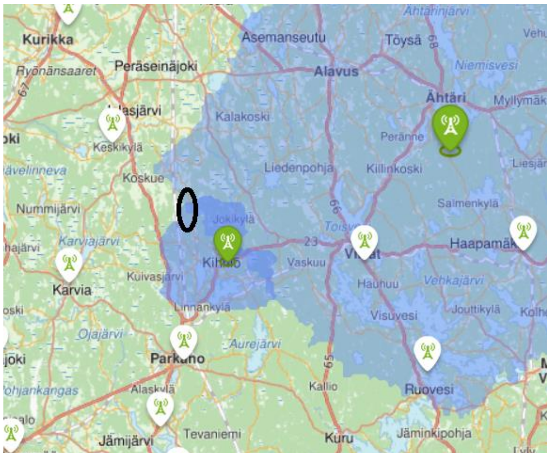
Kuva 8.40. Antenni-tv –vastaanotto Lylyharjun ympäristössä. Kihniön ja Ähtärin lähetasemat on merkitty vihreällä ja Lylyharjun sijainti mustalla merkillä. Sininen väri kuvaa Kihniön ja Ähtärin lähetasemien peittoaluetta.
