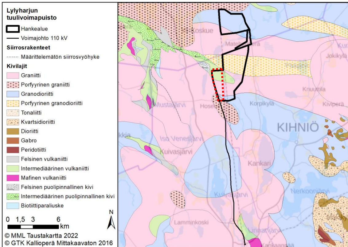
Kuva 8.24. Hankealueen ja sähkönsiirtoreitin kallioperä (Geologian tutkimuskeskus 2021). Kaava-alueen rajaus punaisella katkoviivalla.
