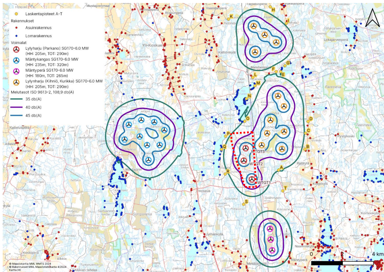
Kuva 8.47 Yhteismallinnuksen tulos, kun huomioidaan Lylyharjun tuulivoimahankkeen kaikki suunnitellut voimalat sekä Mäntyperän ja Mäntykankaan tuulivoimahankkeiden suunnitellut voimalat. Parkanon osayleiskaava-alueen raja- aus on esitetty kuvassa punaisella pisteiviivalla.
