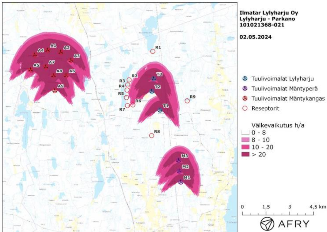
Kuva 8.48 Todennäköinen vuotuinen välkevaikutus, kun mallinnuksessa huomioidaan Parkanon osayleiskaava-alueen voimalat sekä Mäntyperän ja Mäntykankaan tuulivoimahankkeiden voimalat (AFRY 2024).
