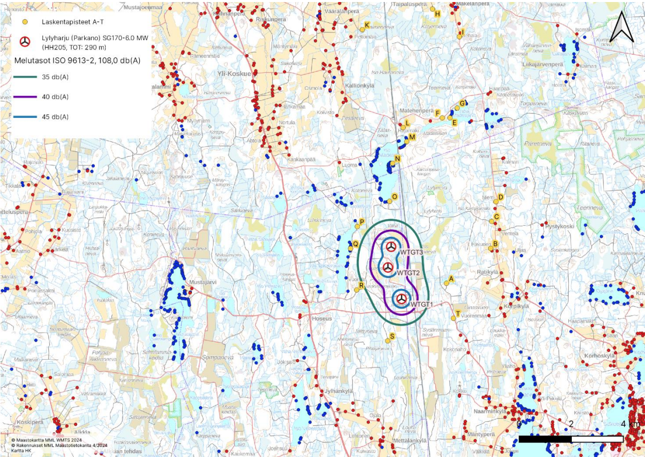
Kuva 8.35. Melumallinnuksen tulos Parkanon osayleiskaava-alueelle suunnitellulla voimalasijoittelulla. Tuulivoimaloiden napakorkeus on 205 metriä ja lähtömelutaso L_{W,A} = 106,0 + 2,0 dB. Karttaan on merkitty havainnointipisteet kirjaimilla A-T.
