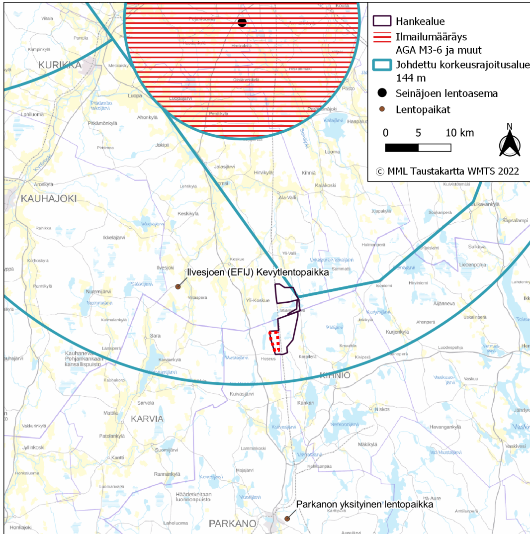
Kuva 8.39. Koko hankealue kuuluu 144 metrin korkeusrajoitusalueelle Seinäjoen lentoaseman vuoksi. Kaava-alueen rajausta punaisella katkoviivalla.
