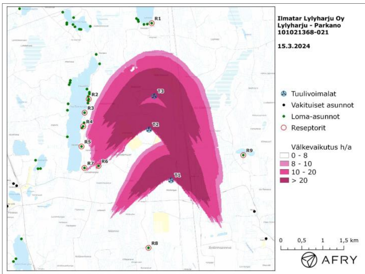
Kuva 8.37. Tuulivoimaloiden aiheuttama todennäköisen välkkeen määrä ilman puuston vaikutusta Parkanon osayleiskaava-alueen voimaloiden osalta (AFRY 2024).
