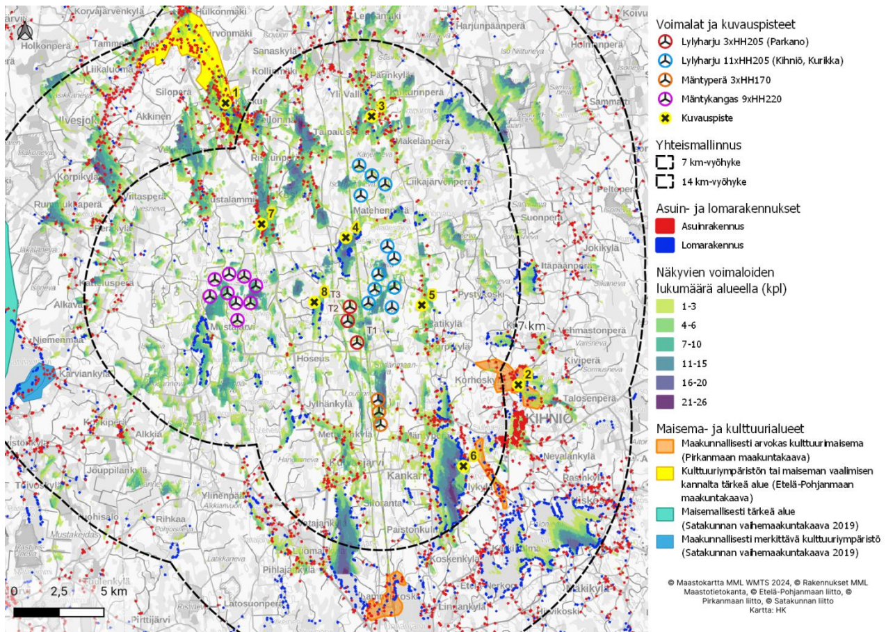
Kuva 8.43 Näkymäalueanalyysi yhteisvaikutuksista Lylyharjun, Mäntyperän ja Mäntykankaan voimaloilla.
