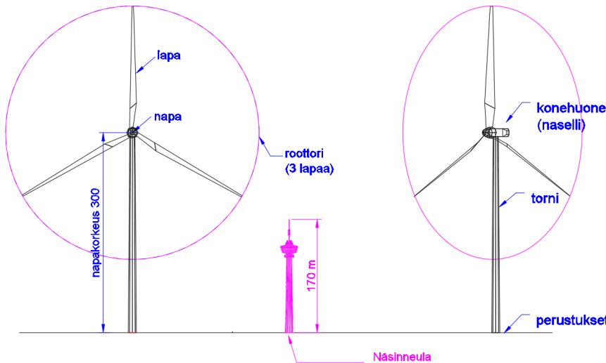
Kuva 1: Tuulivoimalan mittasuhteita ja osien nimityksiä.
